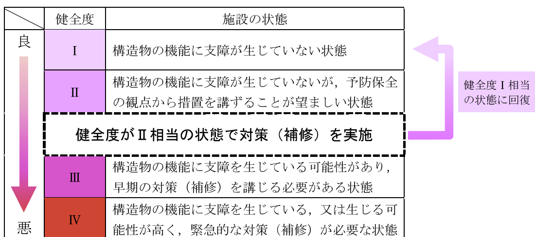
図1-4 トンネルの健全度判定区分と維持管理水準
