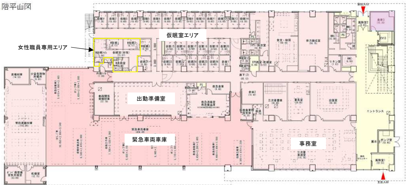
2階平面図
