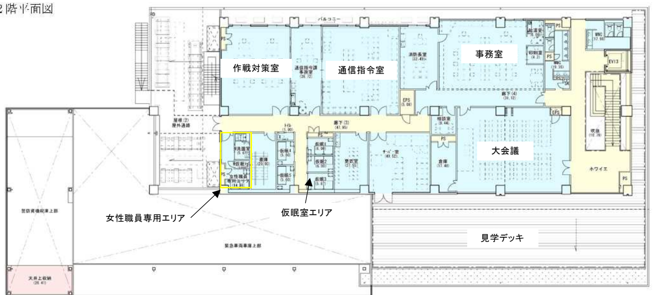
2階平面図
